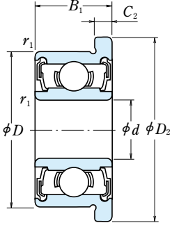
Contact Sealed Type DD
